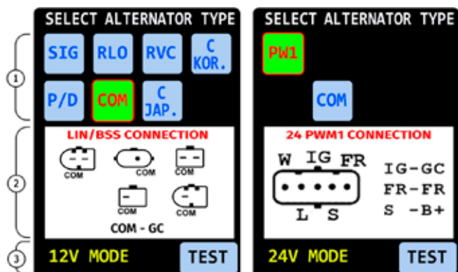
Fig. 6. Tester main menu.
