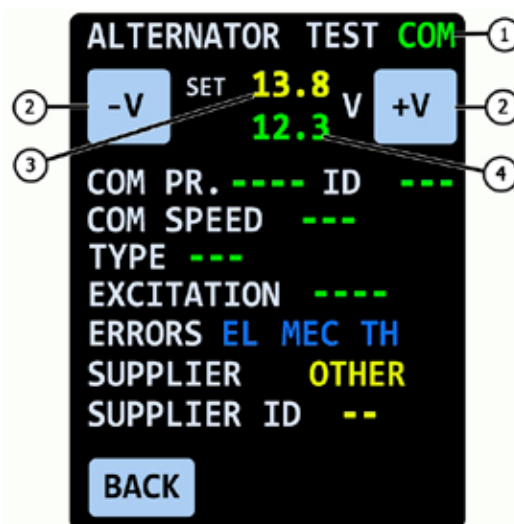
Fig. 7. Pantalla de diagnóstico de alternadores tipo “COM” de 12V.
