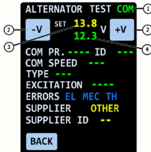
Fig. 7. Tela de diagnóstico de alternadores do tipo “COM” de 12V.
