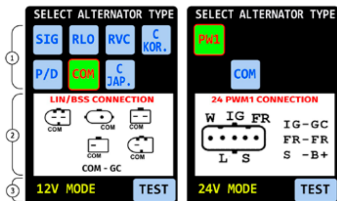
Fig. 6. Menú principal del probador.
