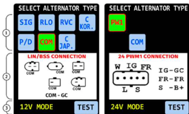
Fig. 6. Menu principal do testador.
