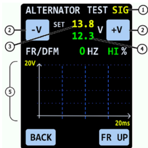
Fig. 9. Tela de diagnóstico de alternadores quando um dos seguintes tipos de alternadores é selecionado: “SIG”, “RLO”, “RVC”, “C KOR.”, “P/D”, “C JAP.”
