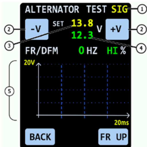
Fig. 9. Pantalla de diagnóstico del alternador cuando se selecciona uno de los siguientes tipos de alternadores: "SIG", "RLO", "RVC", "C KOR.", "P/D", "C JAP."
