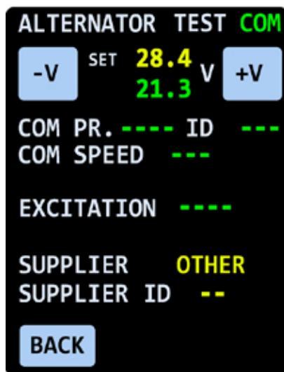
Fig. 8. Tela de diagnóstico de alternadores do tipo "COM" de 24V.
